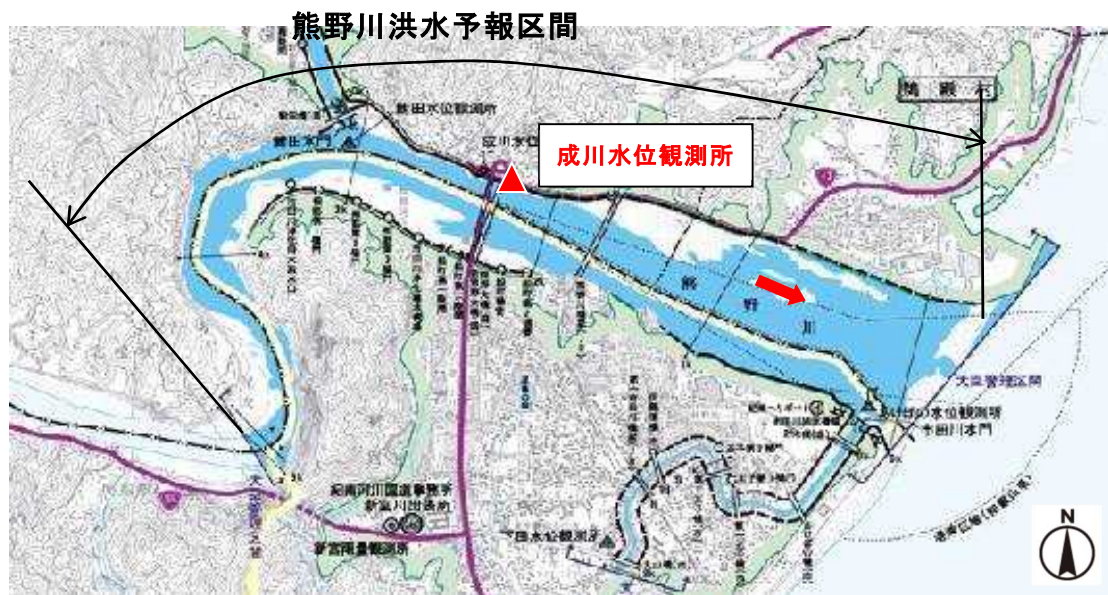
図-2.9 新宮川水系洪水予報実施区域
