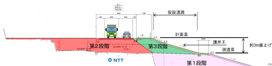
標準断面図(日足地区)
