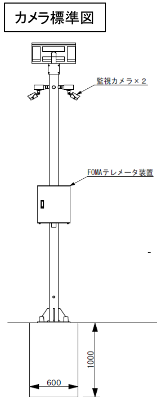
カメラ詳細図
