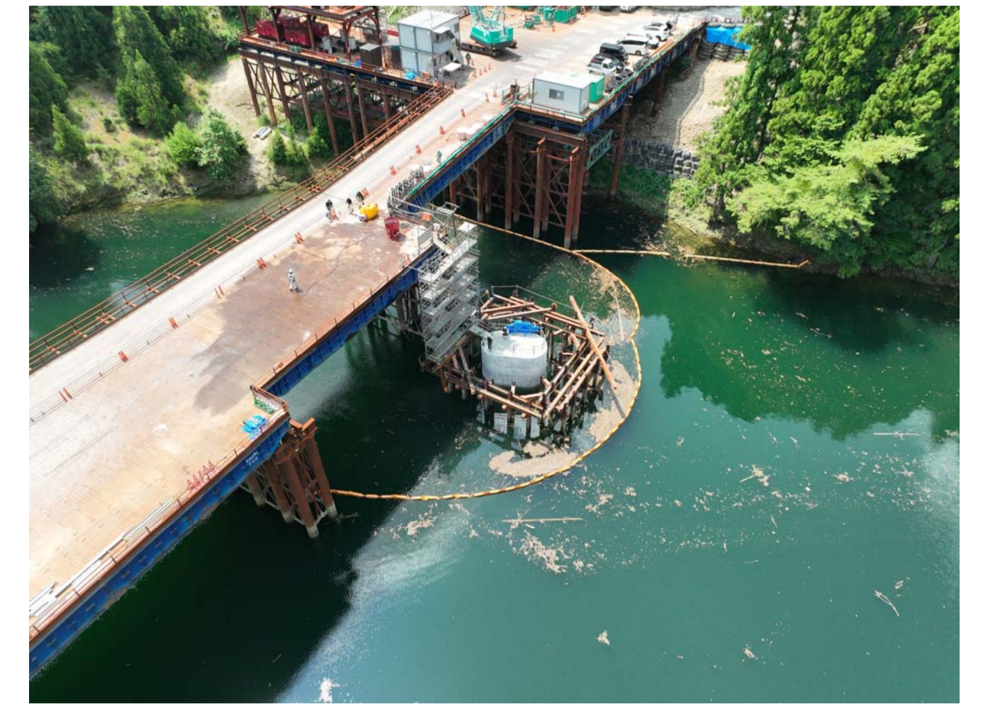
④ 北山村下尾井(1号橋)
