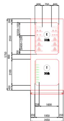
神戸第3共同溝 標準断面図 (施工難易度：B30mm)
