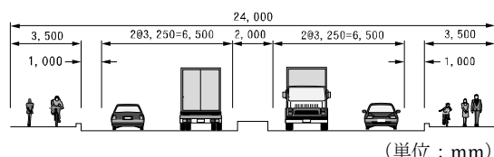
標準断面図
