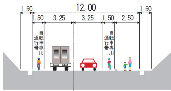
標準断面図
