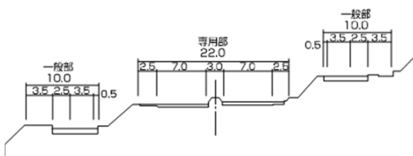
標準断面図
