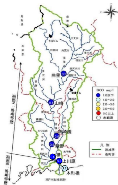
図 1.5.7 BOD (75%水質値)
