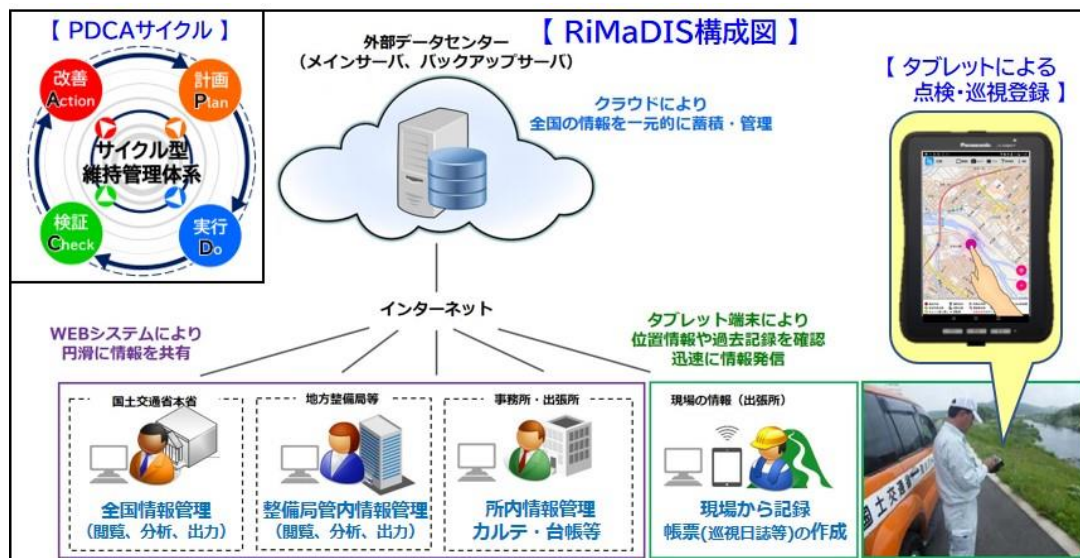
図 5.1.1 RiMaDIS 構成図
