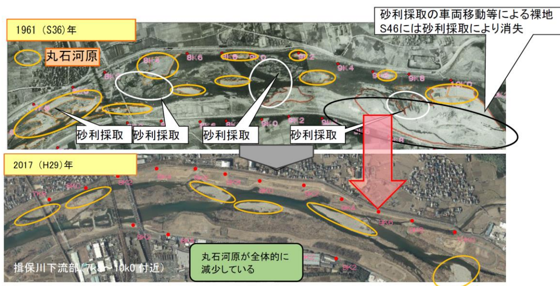
図 1.3.3 揖保川 横断形・丸石河原の変化
