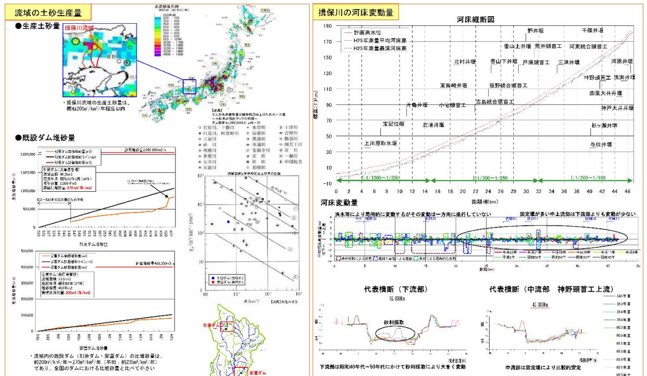
図 1.4.1 揖保川流域の土砂動態
