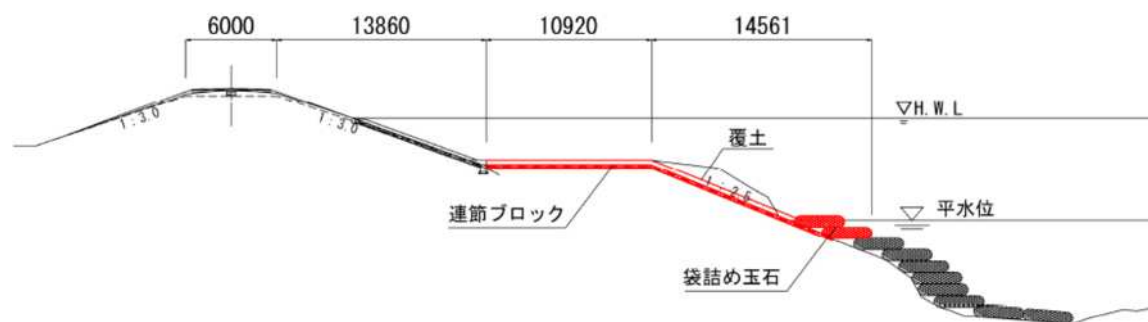
標準断面図
