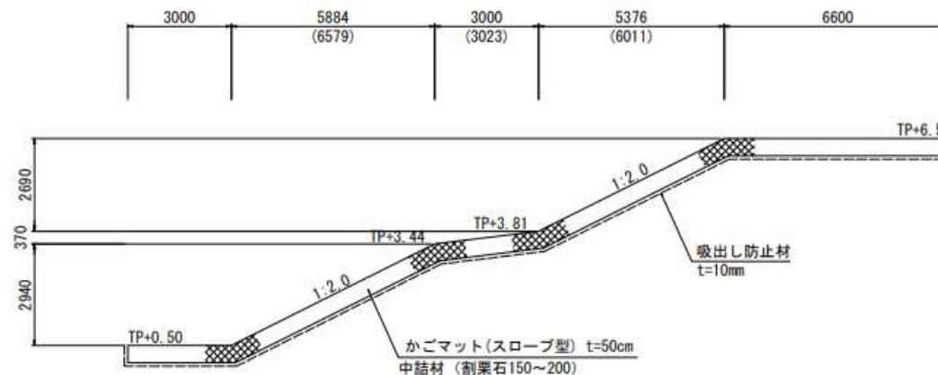
標準断面図
