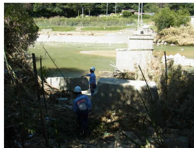
被災状況調査(焼野1号橋)
