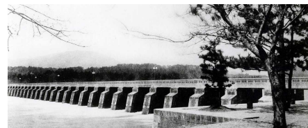
南郷洗堰
